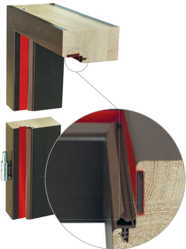
klesajúce tesnenie naspodu krídla (verzia 2)
