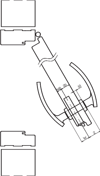
VLOŽKY HEKTOR PRE KRÍDLA FOGO
