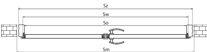
LIŠTA 60 mm (L/MF) / 80mm (L/M8)
