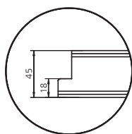
rez dverí
