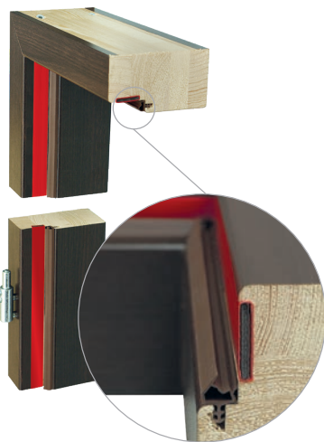
klesajúce tesnenie naspodu krídla (verzia 2)
