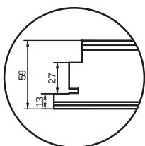
rez dverí
