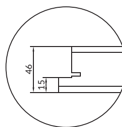
rez dverí
