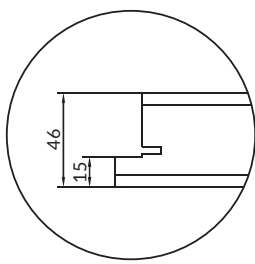
rez dverí
